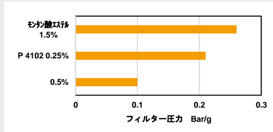
事例4. 酸化チタン50%添加PBT フィルター圧力低減
