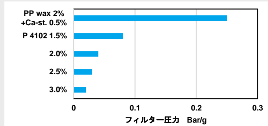
事例3. 酸化チタン70%添加ポリプロピレン フィルター圧力低減
