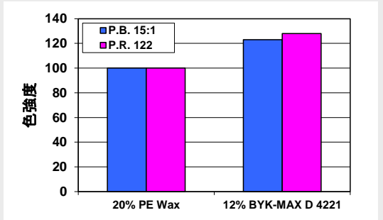
事例2. 有機顔料40%添加LDPE 着色性向上
