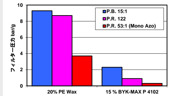
事例1. 有機顔料40%添加LDPE フィルター圧力(ISO 23900-5)低減
